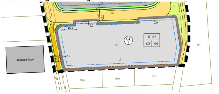
Planzeichnung 1. Änderung M1: 1.000
